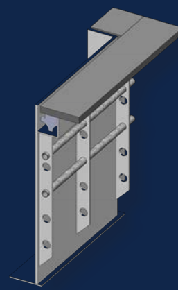
Type 2 Overflow direct over de zwembadrand
