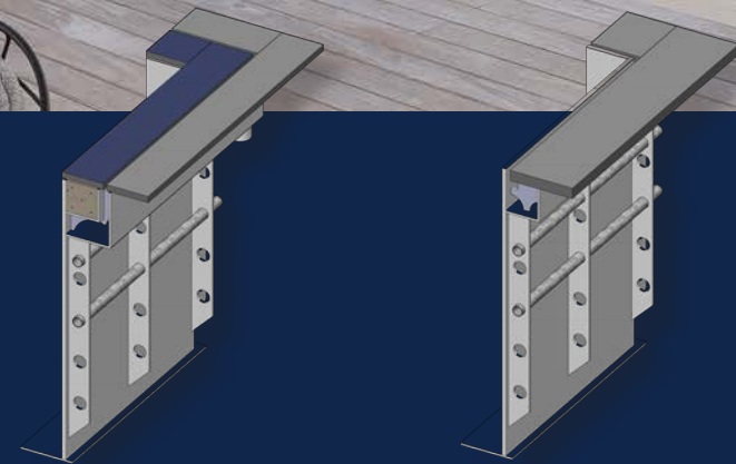
Type 1 Overflow avec margelle immergée
